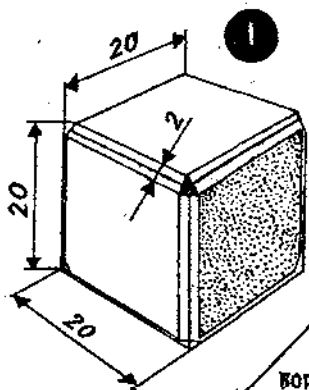
УГЛОВОЙ КУБИК
